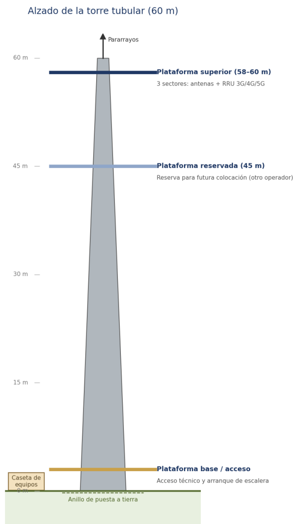
Figura 1. Alzado esquemático de la torre tubular (60 m).
